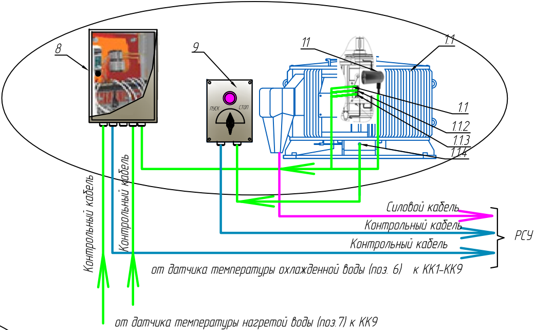
Узел "А"(для КК1-КК9)
