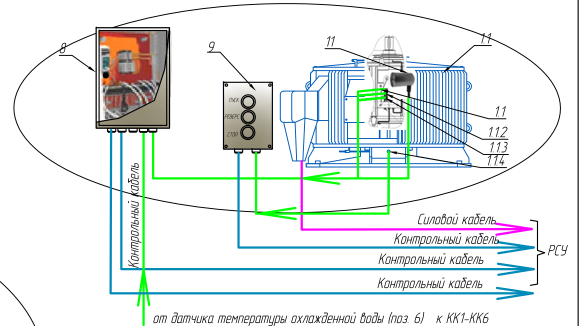
Узел "А"(для КК1-КК6)
